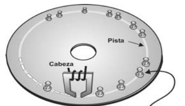
Campos magnéticos inducidos en el disco por la cabeza de escritura, a manera de clavitos magnéticos para memorizar bits de datos.
