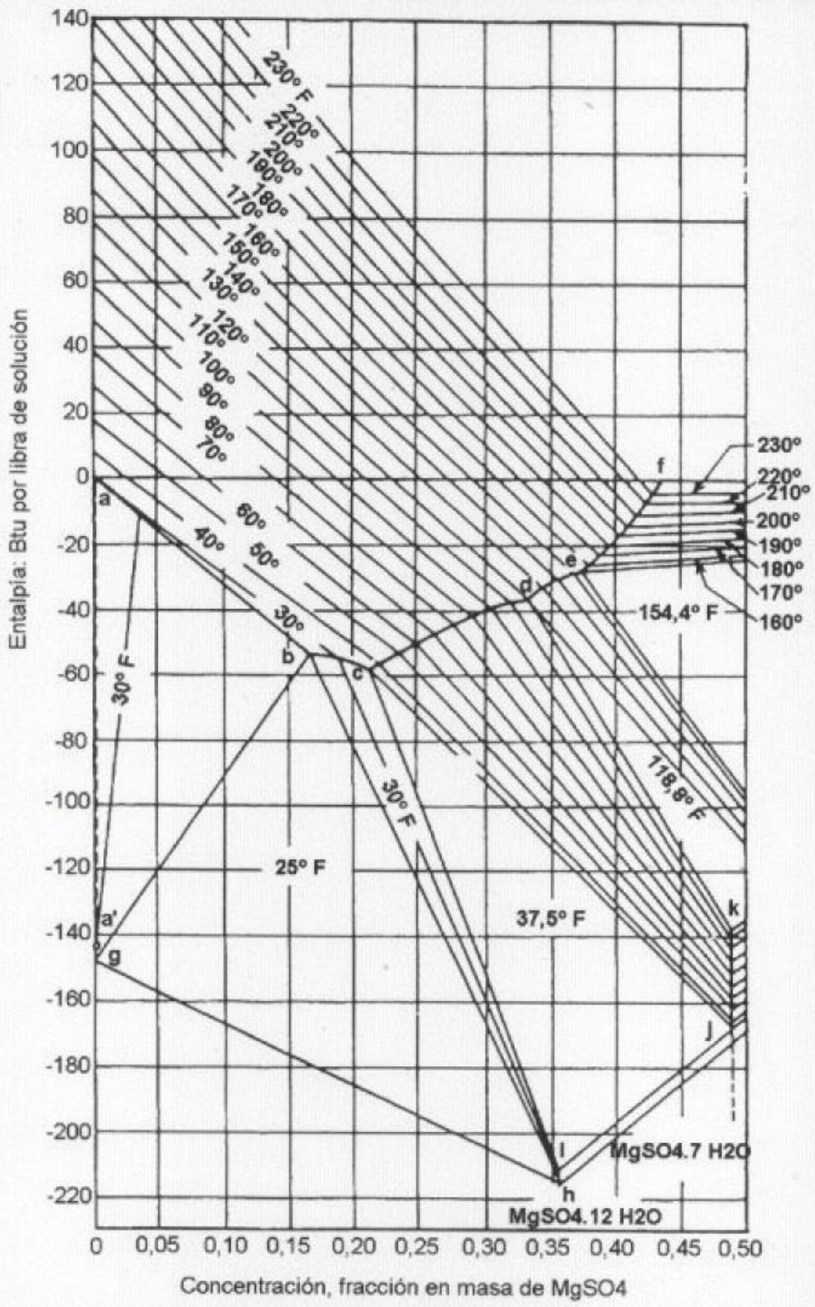
Diagrama entalpía concentración para el sistema sulfato de magnesio – agua. Estado de referencia: sulfato de magnesio y agua a 32° F y a la presión de vapor del agua
