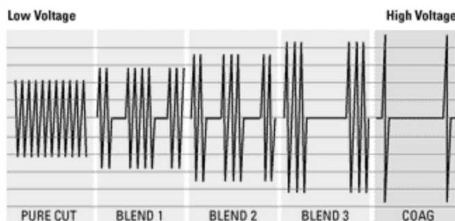
Fig.3 Señales utilizadas en los diferentes procesos [1]
