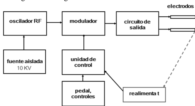
Fig.1 Diagrama de bloques del Electrobisturí [3]
