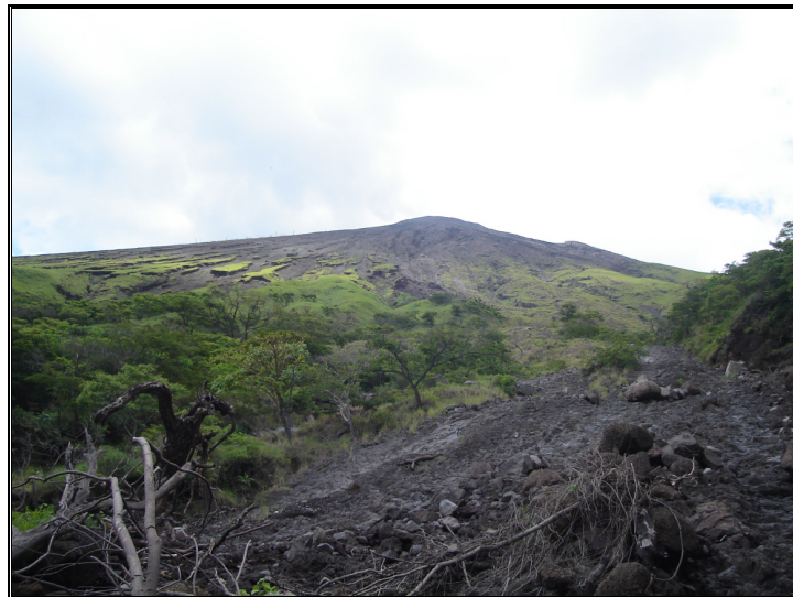
Fotografía 3. Área fuente de escombros para los lahares. Ladera Sur del Volcán San Cristóbal
