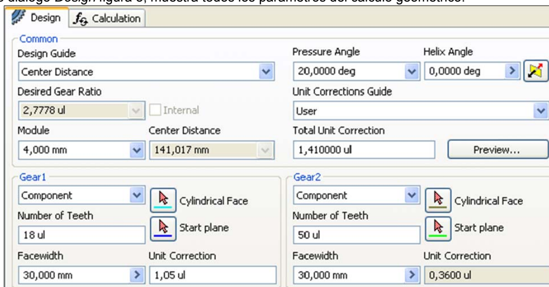
Figura 3. Caja de diálogo Design.
